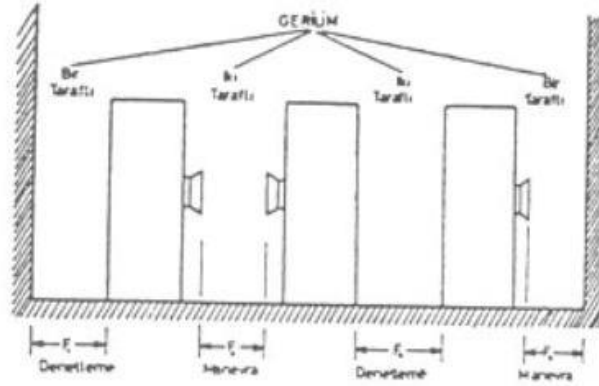
Şekil - 1 Hücre cephelerinin tel kafes kapı ve dolu duvar olması durumunda geçit genişlikleri
