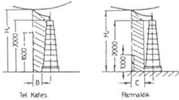
Şekil-4 Tesis içerisindeki koruma alanı ve en küçük yükseklik ( H_1 )
