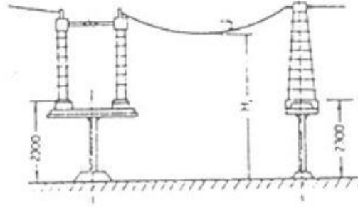
Şekil-3 Tesis içerisinde çitle çevrilmemiş yürünülen yüzeyler üzerindeki iletkenlerin yerden yükseklikleri (Çizelge-3'e göre).
