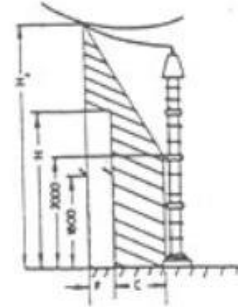
Şekil-7 Yere konulan ve geçitli normal çiti bulunan aygıtlarda koruma alanı
