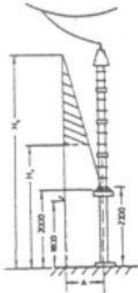
Şekil-5 Dayanak (mesnet) üzerindeki aygıtlarda koruma alanı
